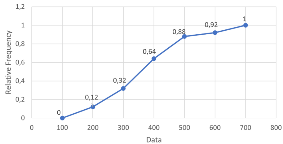
Ogive
